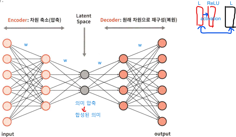
[그림 10-1] 오토인코더의 구조
